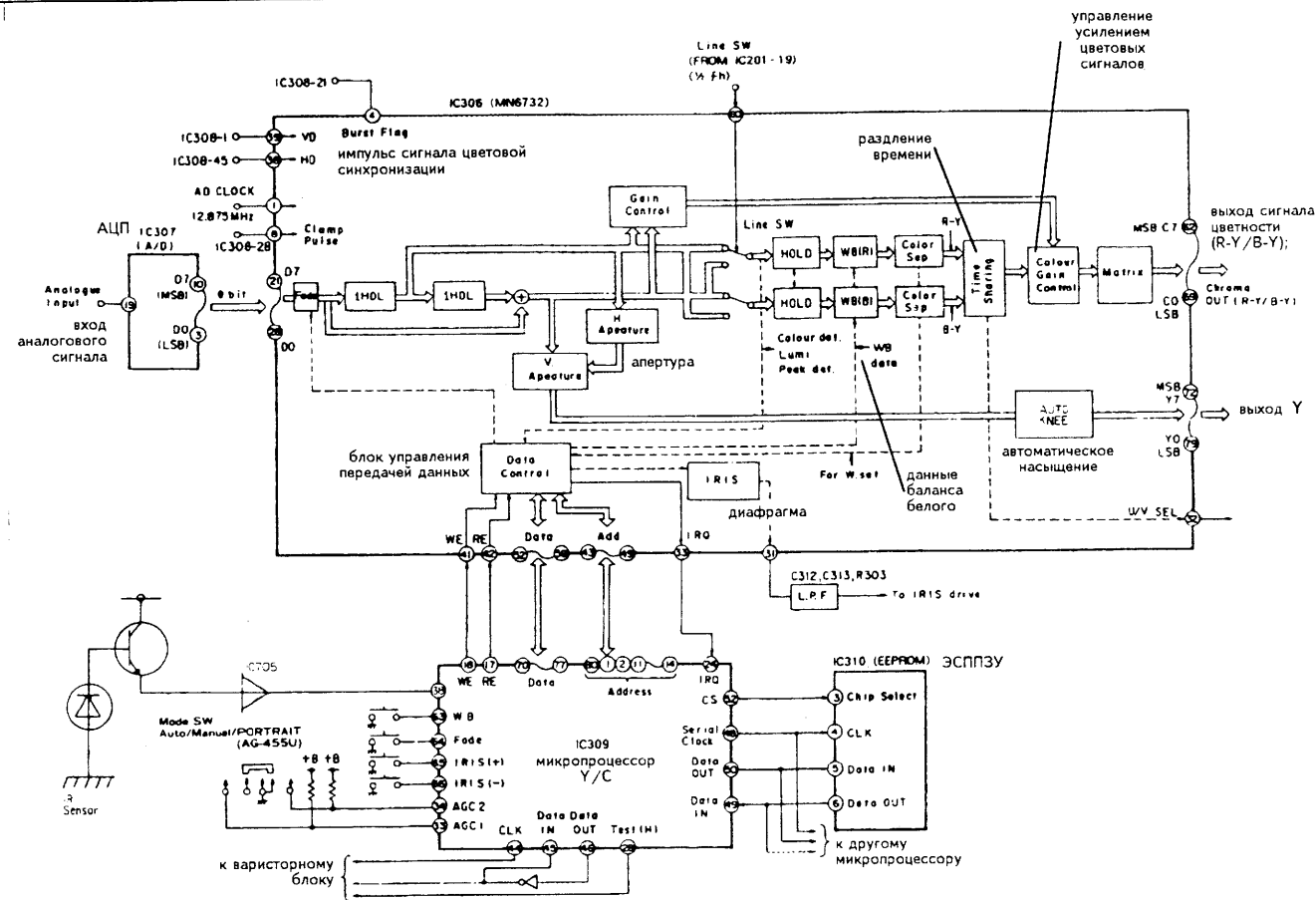
Рис. 3-4 Упрощенная структурная схема обработки сигнала Y/C:
