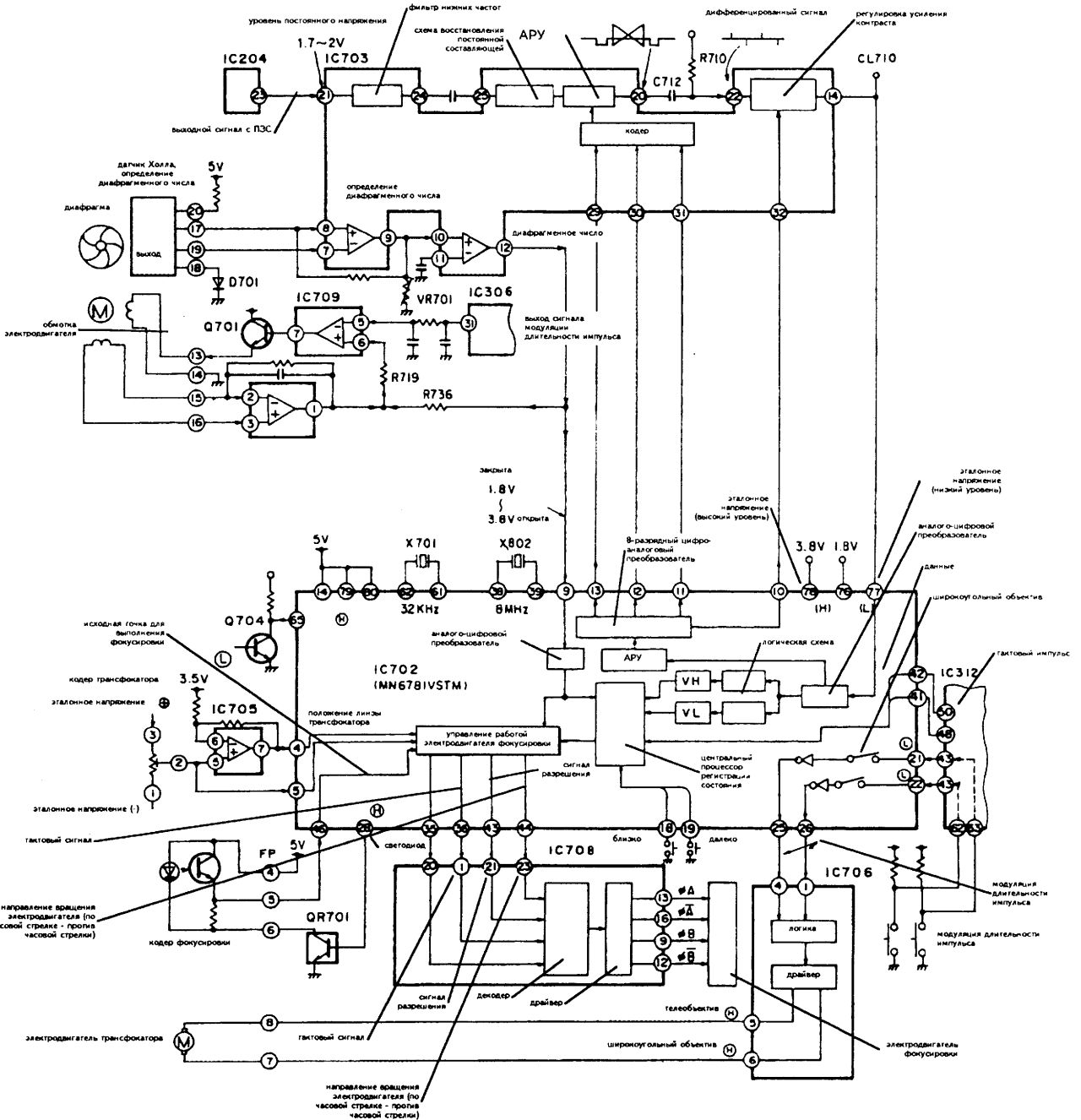
Рис. 4-13. Блок схема системы цифровой автоматической фокусировки с компьютерным управлением
